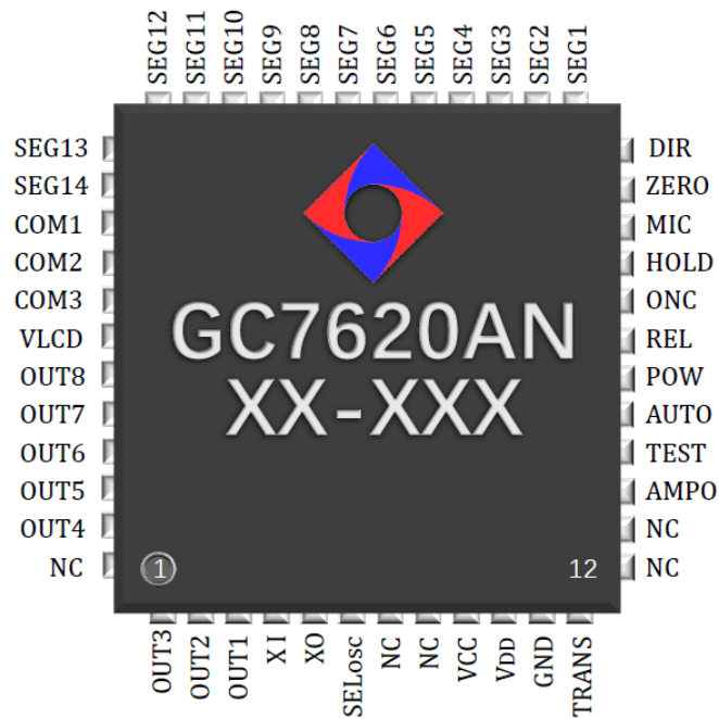
QFN48 脚的封装片管脚图
