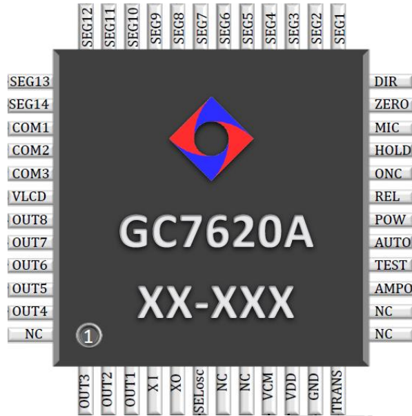
LQFP48 脚的封装片管脚图
